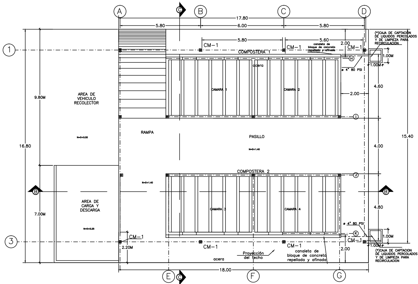
PLANTA DE DISTRIBUCION PLANTEL DE COMPOSTERA Esc. 1:100
